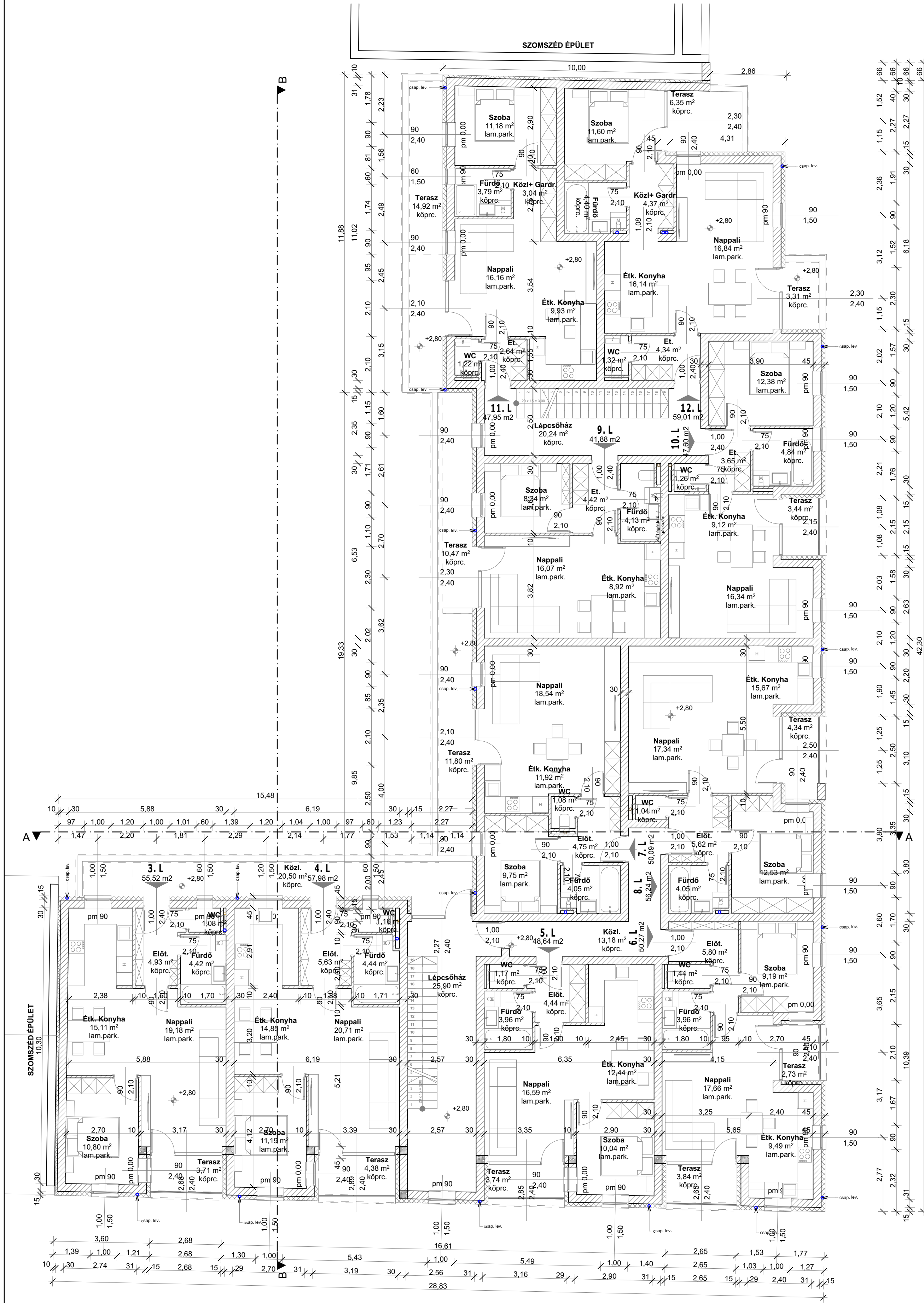
I. EMELETI ALAPRAJZ m=1:100
