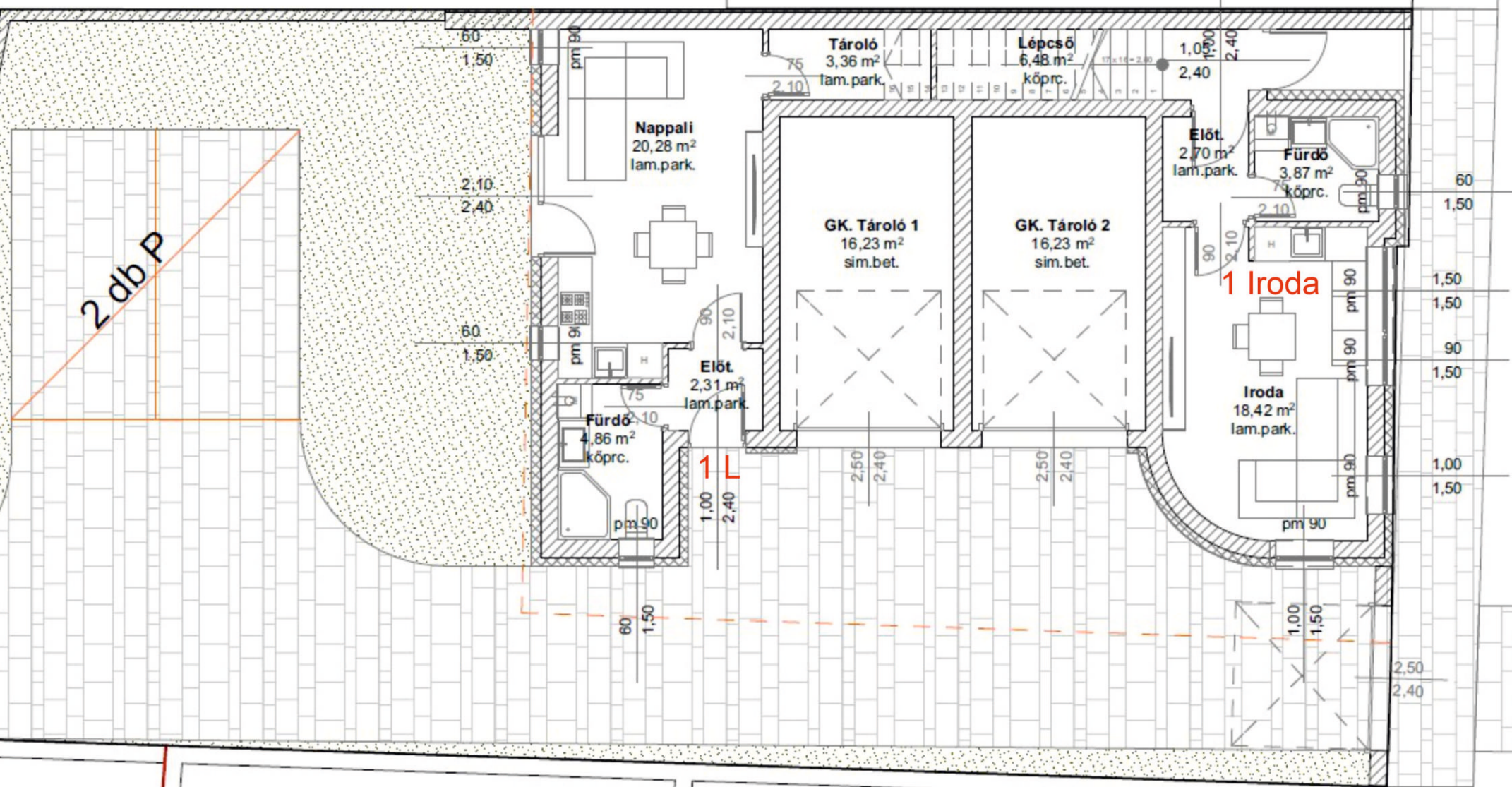
FÖLDSZINTI ALAPRAJZ
