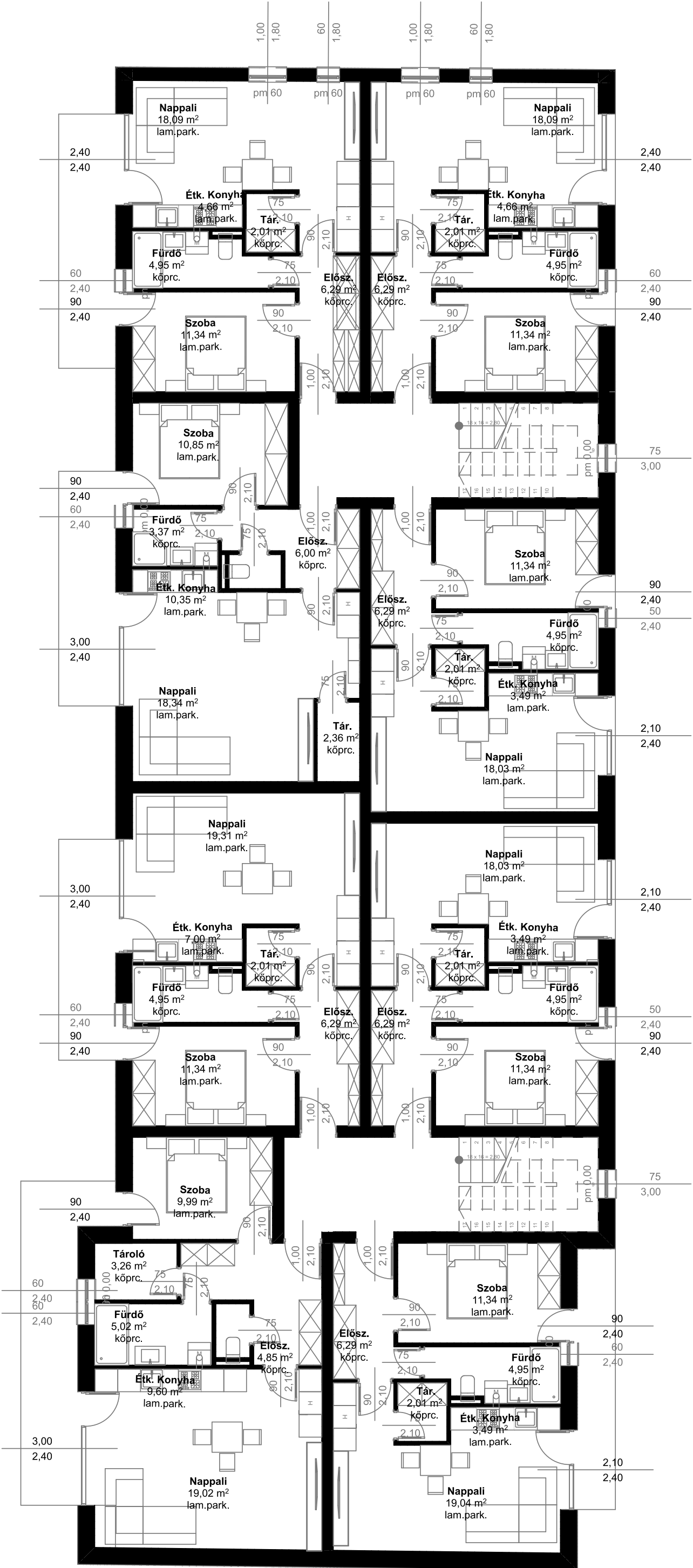
1. EMELETI ALAPRAJZ M=1:100
