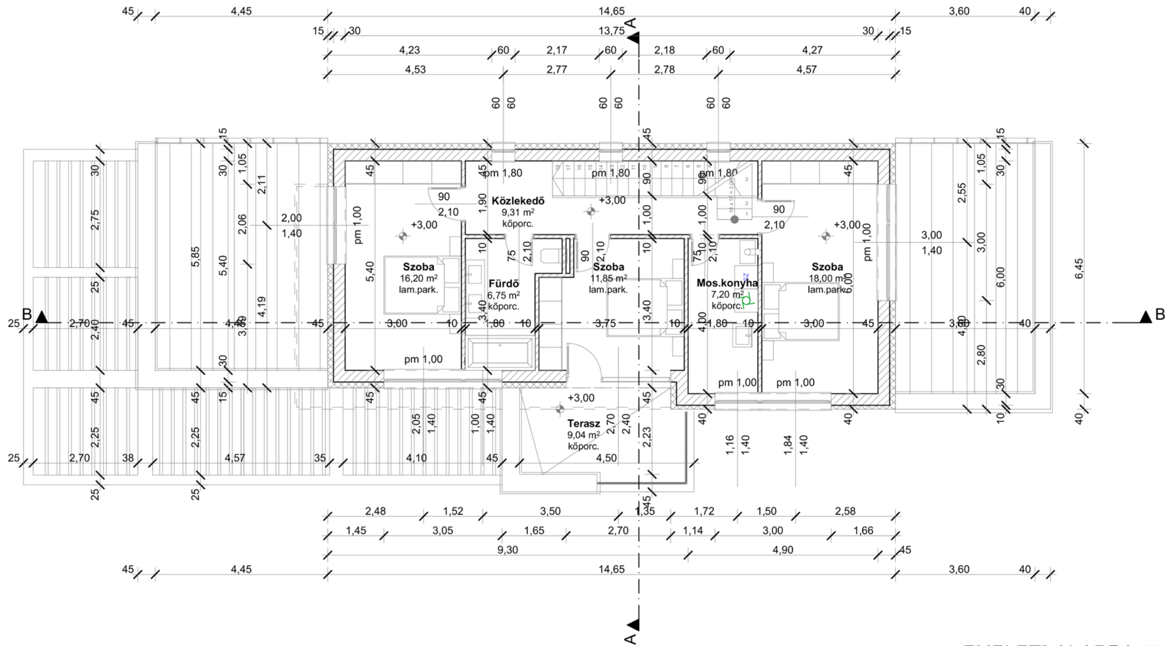
EMELETI ALAPRAJZ m=1:100
