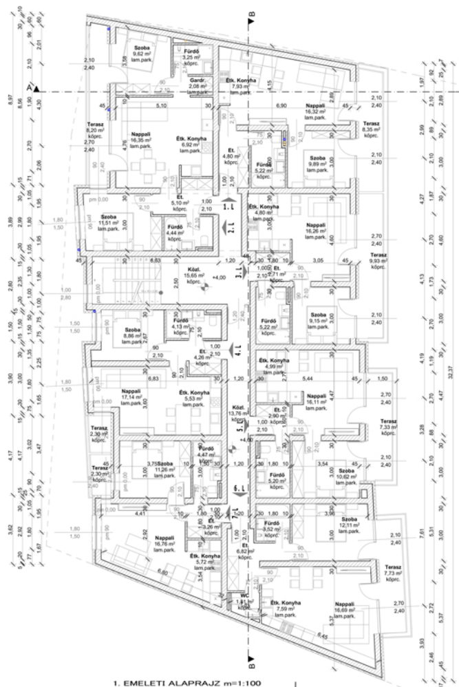
1. EMELETI ALAPRAJZ m=1:100
